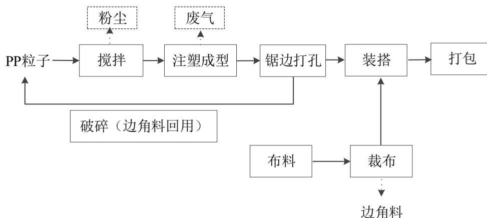
图 2.2.1-3 PP 箱包工艺流程图
