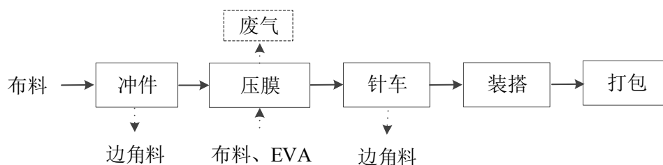
图 2.2.1-2 布箱包工艺流程图
