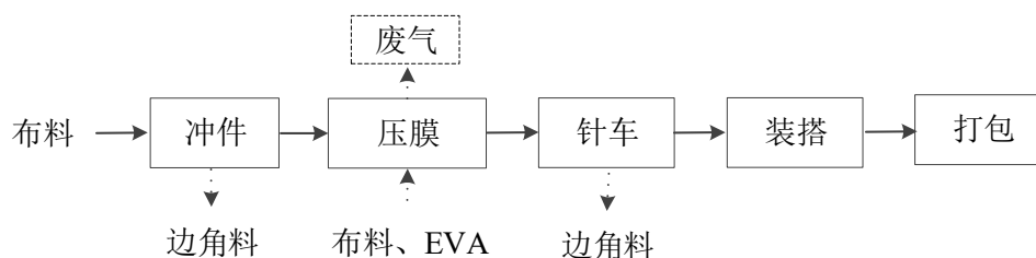
图 2 布箱包工艺流程图
