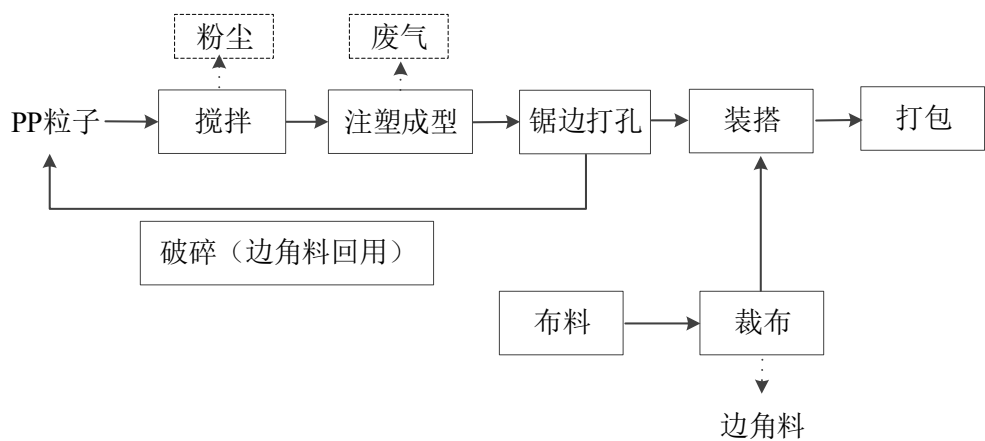
图 3 PP 箱包工艺流程图
