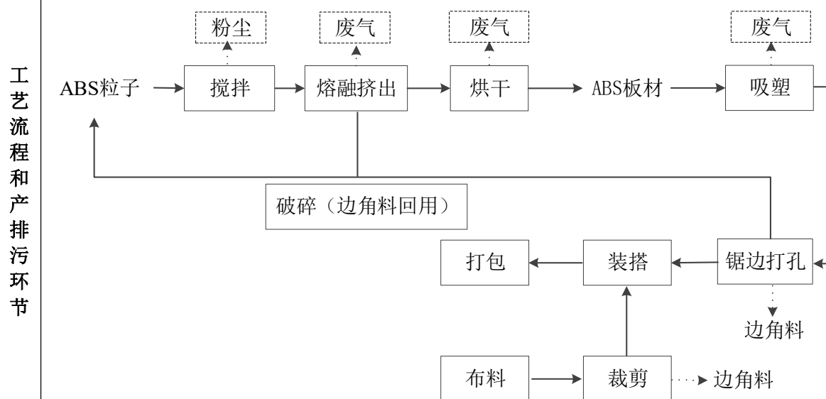
图 2.2.1-1 ABS 拉链箱包生产工艺流程图
