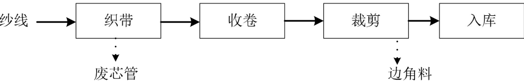
图 2-3 箱包织带工艺流程图
