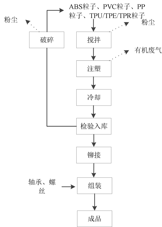
图 2-2 箱包轮子工艺流程图
