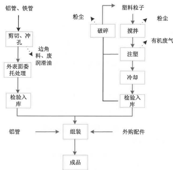
图 1 ABS 箱包生产工艺流程图
