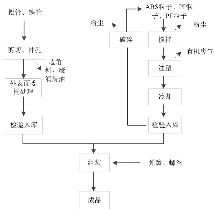
图 2-1 箱包拉杆工艺流程图
