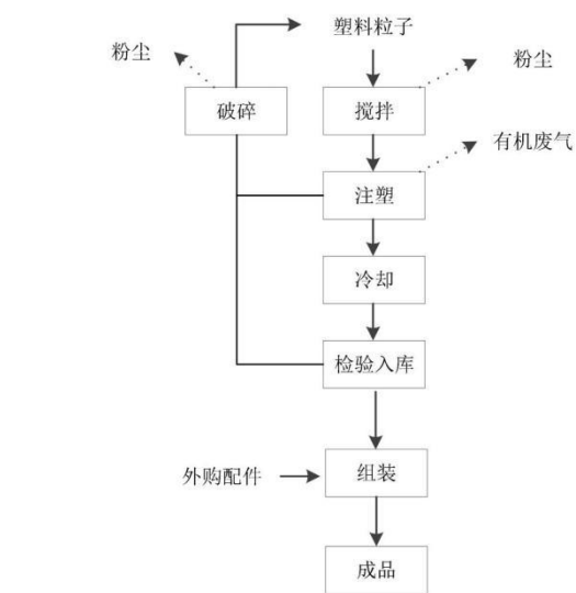
图 2 箱包轮子工艺流程图
