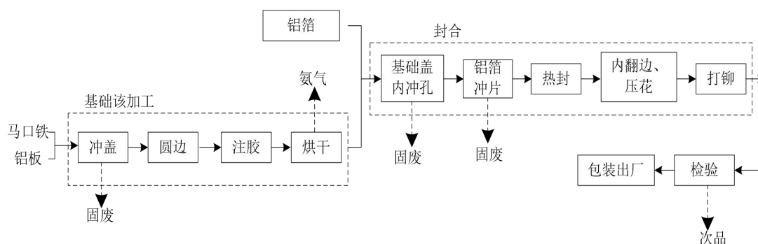
图 2-2 生产工艺流程及产物环节图
