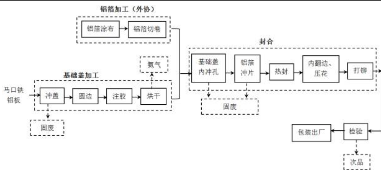
图 2-3 原有工程工艺流程及产污节点示意图
